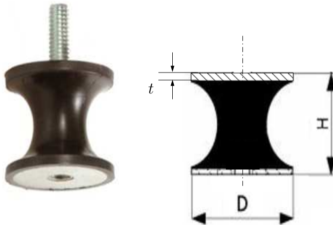
Abbildung 1: Gummi–Rundpuffer
