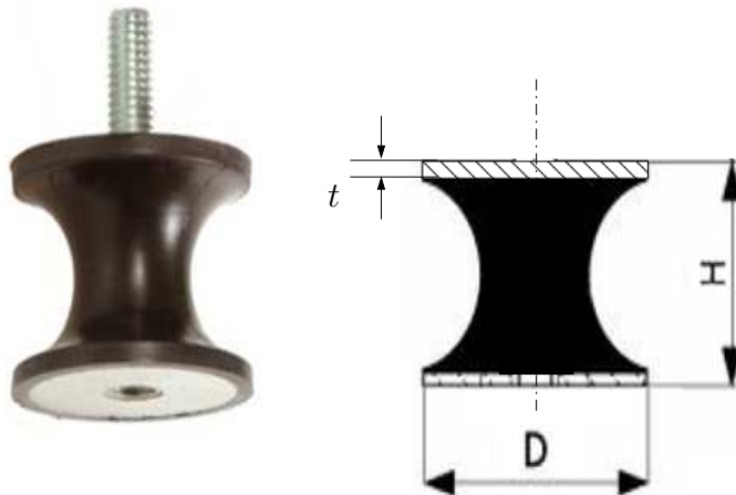
Abbildung 1: Gummi–Rundpuffer
